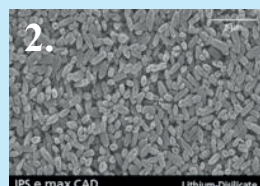
2. Крайно изкристализиране на IPS e.max CAD (темперован при 850° C). Структурата се състои от приблизително 70% финнозърнести литиум дисиликат кристалчета, вложени в глас-матрица. Посредством ецване с течнокиселинна пара глас-фазата се разтваря и литиум дисиликатните кристалчета стават видими.
